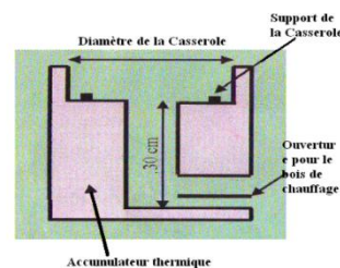
Fonctionnement de Rocket LORENA STOVE: Utiliser ce foyer amélioré pour sauvegarder l'énergie et l'environnement.
